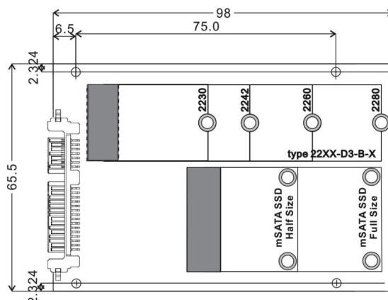
外型尺寸 (單位:mm)
